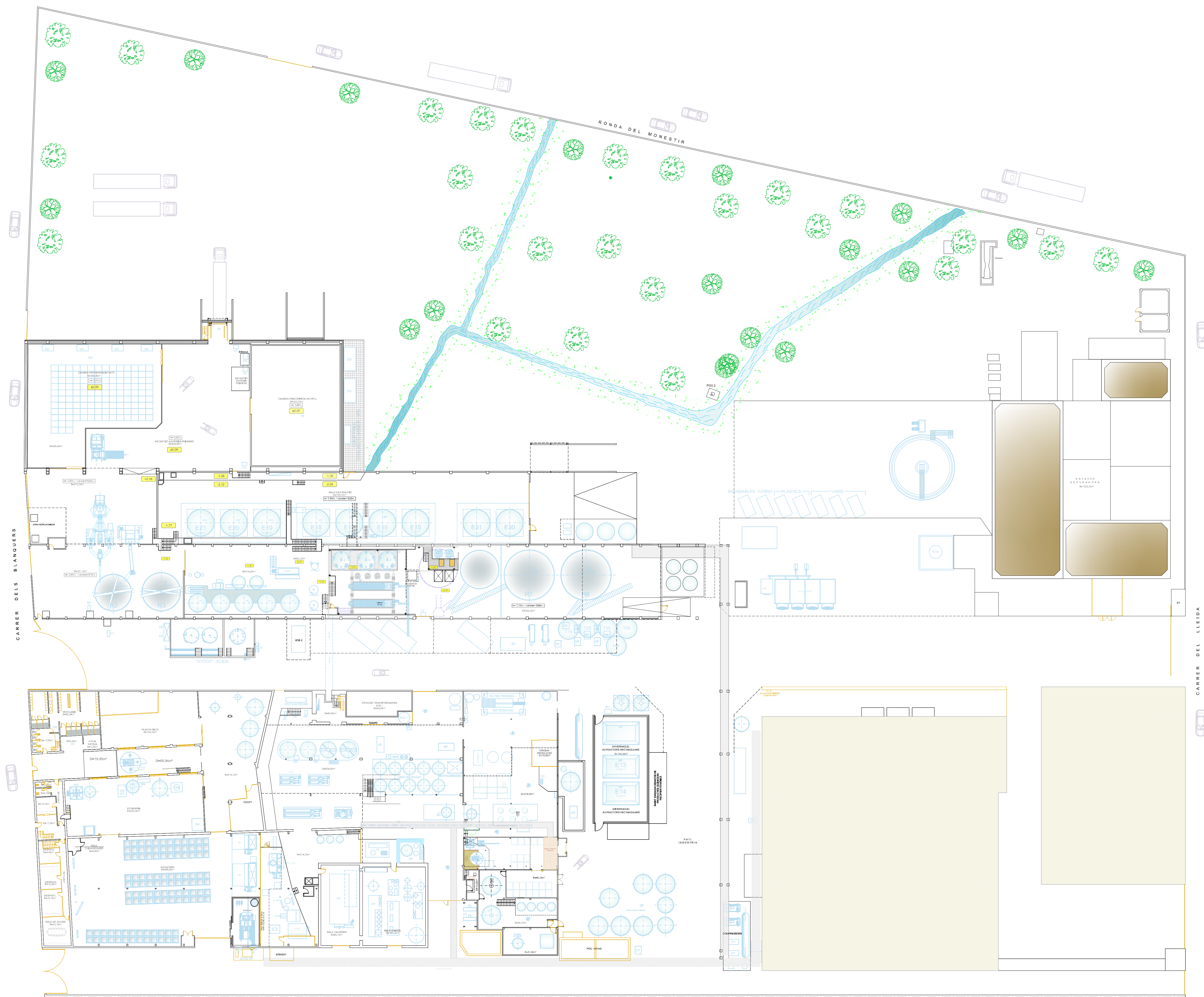
PLANTA BAIXA E: 1/300
