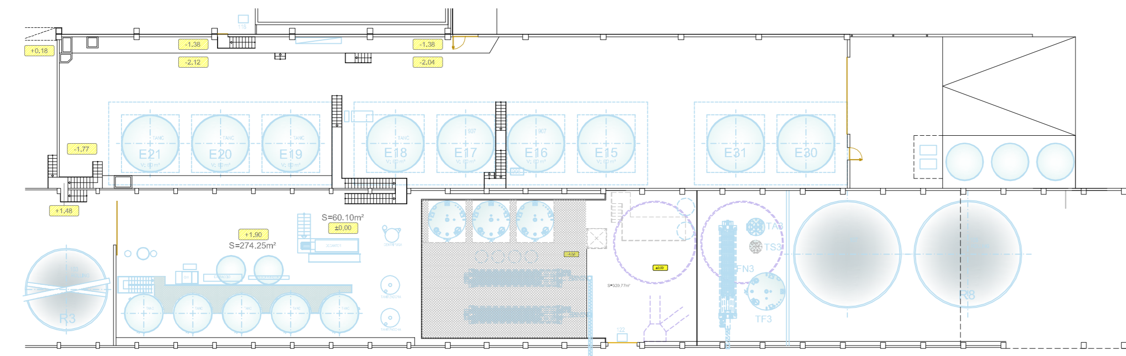
PLANTA ALTELL (nivell +4,00) E: 1/300
