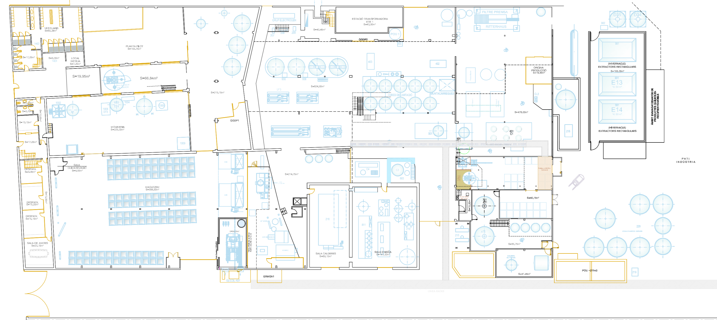
PLANTA BAIXA E: 1/300
